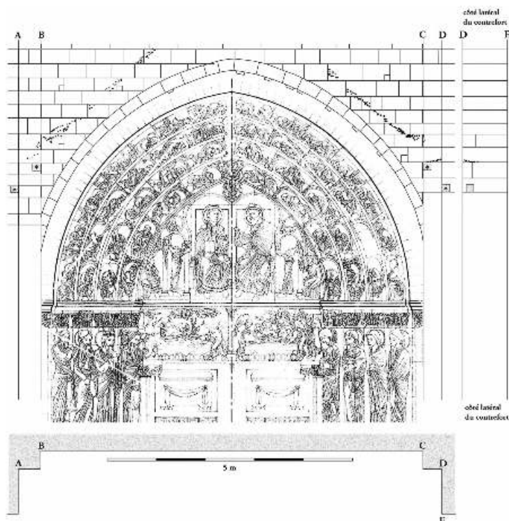
Fig. n°1 : Senlis « Porte ouest de la Cathédrale Notre-Dame ». Portail occidental : relevé pierre à pierre du mur de façade supérieur au tympan (relevé Poncelet). Traces de bûchage au niveau du passage en bâtière de la toiture au-dessus de l'arc. Deux encoches de fixation de poutrelle de la charpente sur les côtés latéraux internes des contreforts (grisé) (Relevé et dessins G.-P. Woimant, CG de l'Oise)
